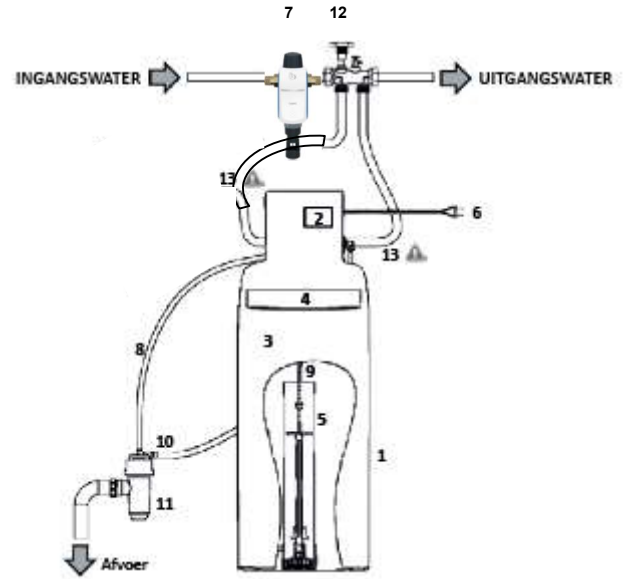
^ Principeschema
